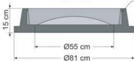
Vista corte
